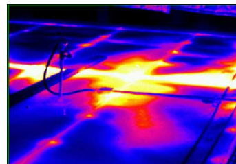
Odkrivanje vlage na ravni strehi
