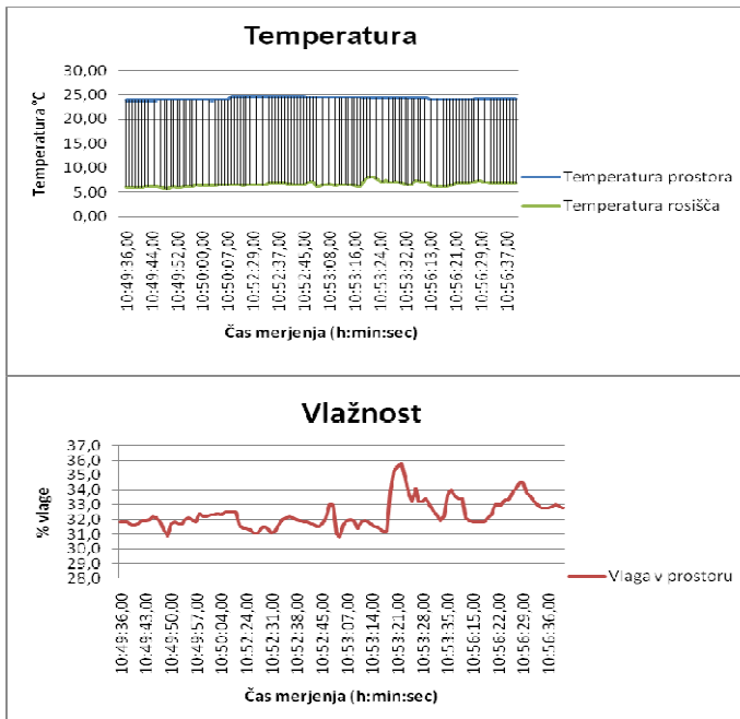
Sprememba vlage, temperature in temperature rosišča v odvisnosti od časa
