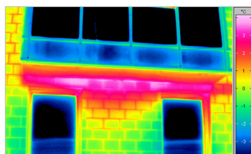
Odkrivanje toplotnega mostu
