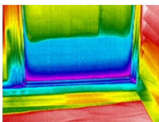
Odkrivanje slabe zatesnitve oken
